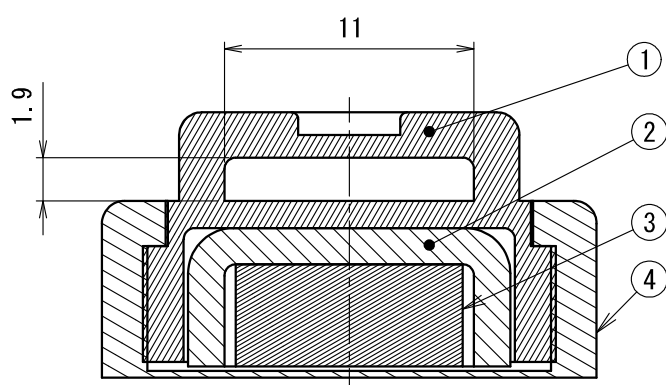
断面 A-A
